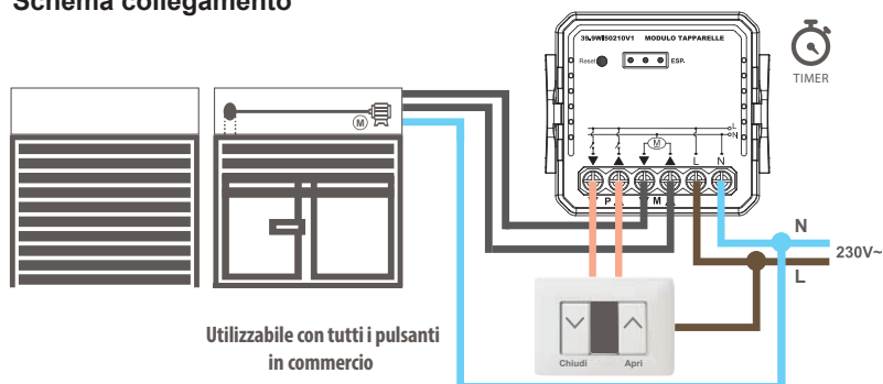
Schema collegamento
